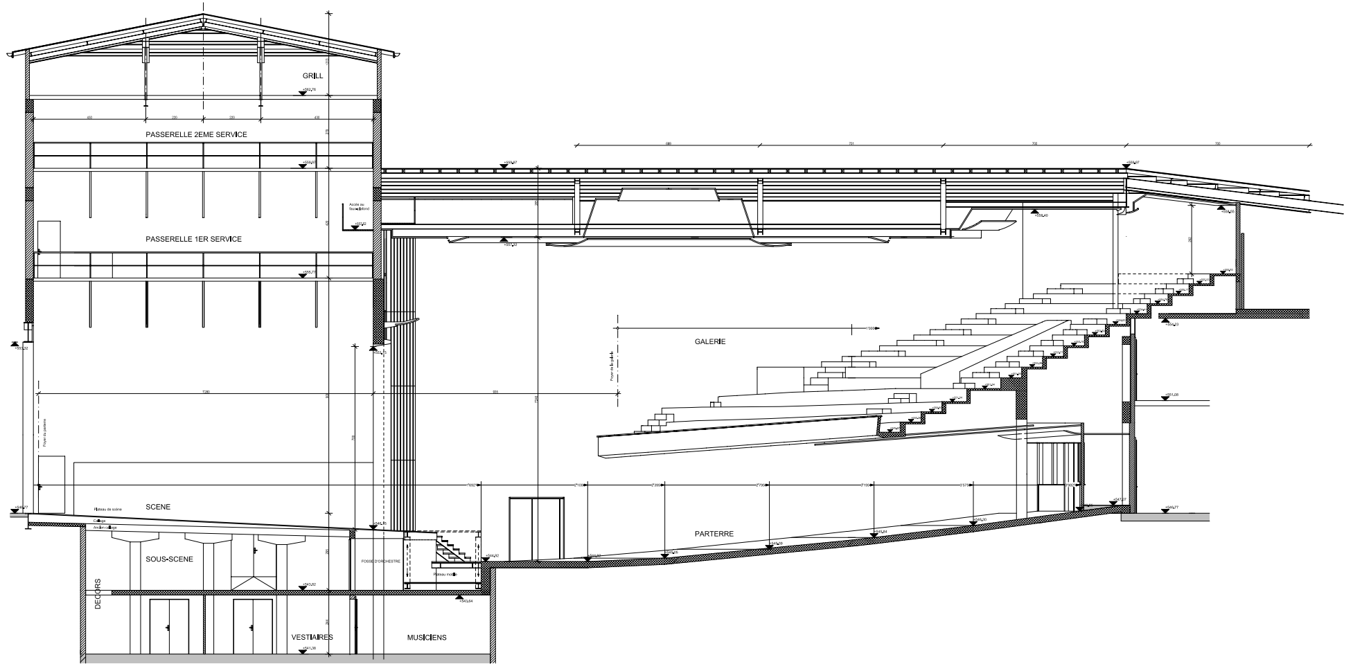
COUPE BB
