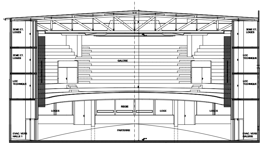
COUPE CC
