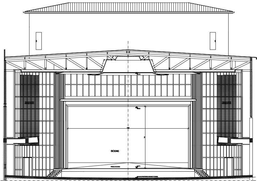
COUPE BB
